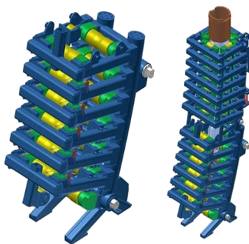
VODÍCÍ VÁLEČKOVÝ SEGMENT D 470 MM
